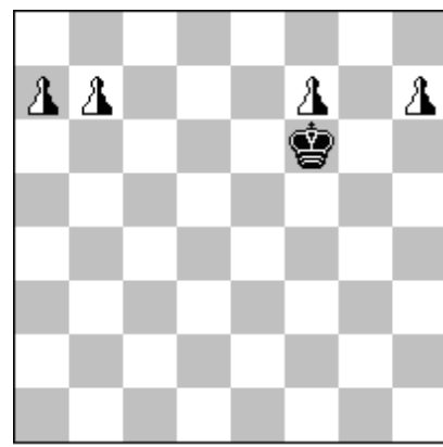
h # 11 (0 + 1 + 4) Couscous circe, Einstein
