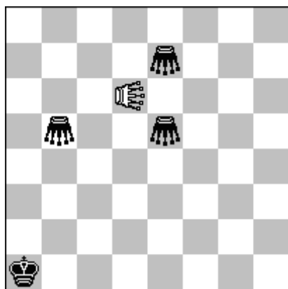
h # 7 3.1.1... (1 + 4) (d6 - contre grasshopper)
